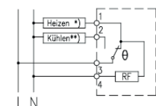
TWR 60 Umschalter (CO) mit thermischer Rückführung
