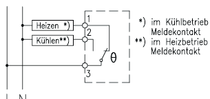
TRW 60 / TKW 60 Umschalter (CO)
